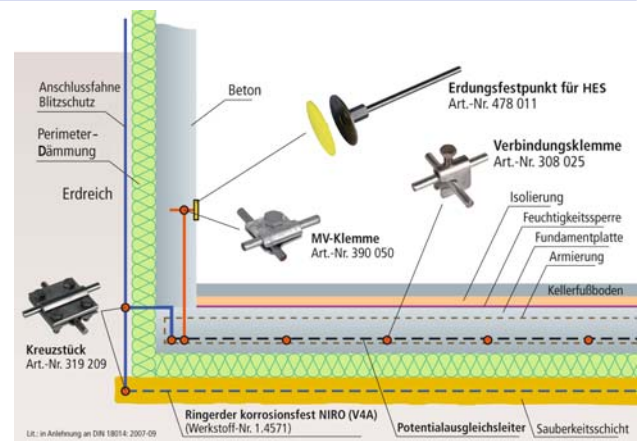
Anordnung des Fundamentertders bei einer Fundamentplatte mit Perimeterdämmung (vollisoliert)
