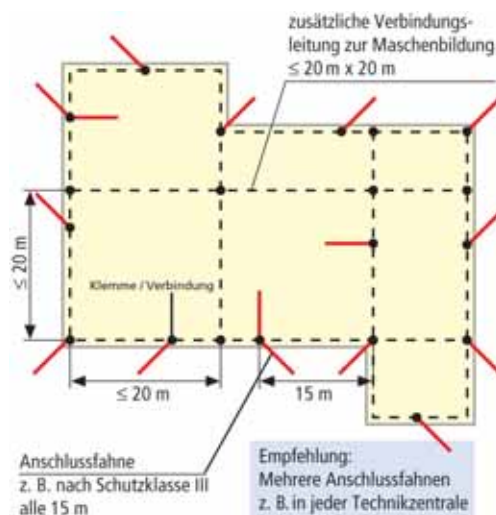
Fundamenterder mit Anschlusssteilen / -fahnen nach innen und außen
