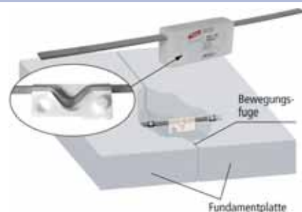
Überbrückungen des Fundamenterders
